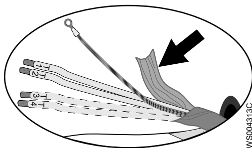
Рис. 10: Медная фольга на проводах цепей контроля.
