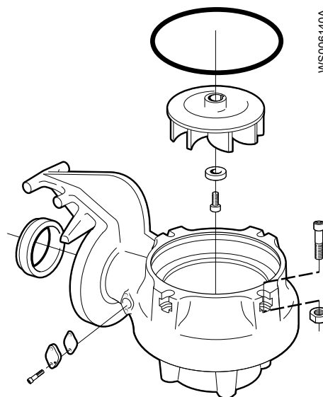
Рис. 14: Рабочее колесо типа D
