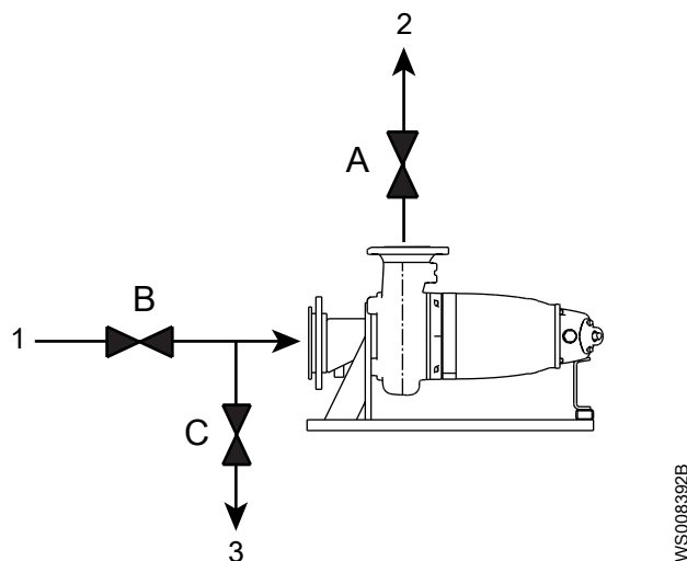
Рис. 21: Клапаны А—D для варианта Т (показаны типовые насосы)
