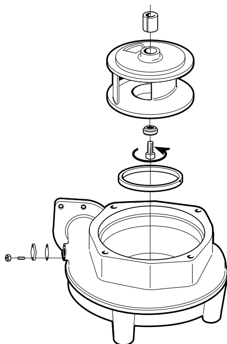
Рис. 10: Рабочее колесо типа C
