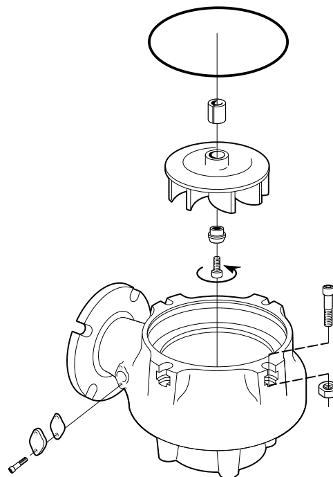
Рис. 11: Рабочее колесо типа D
