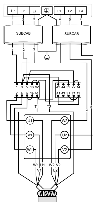
Клеммная колодка и контактный блок
