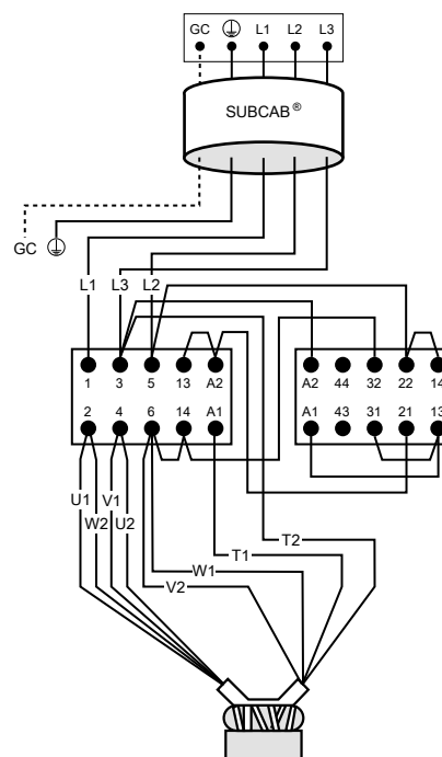
Соединение треугольником
