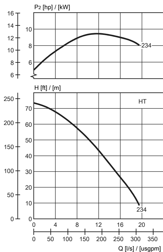
Рис. 16: HT, 60 Гц
