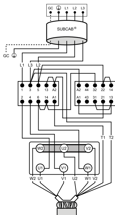
Соединение звездой
