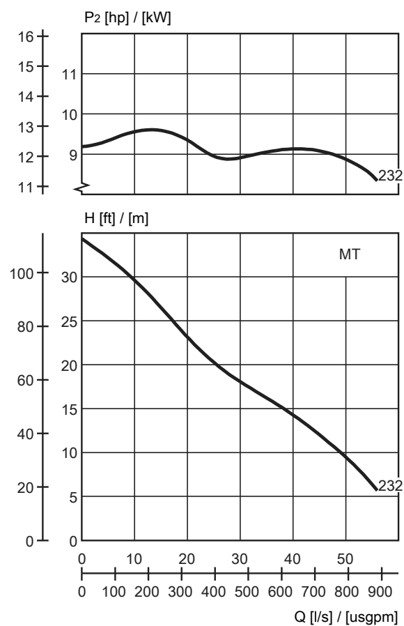
Рис. 14: MT, 60 Гц
