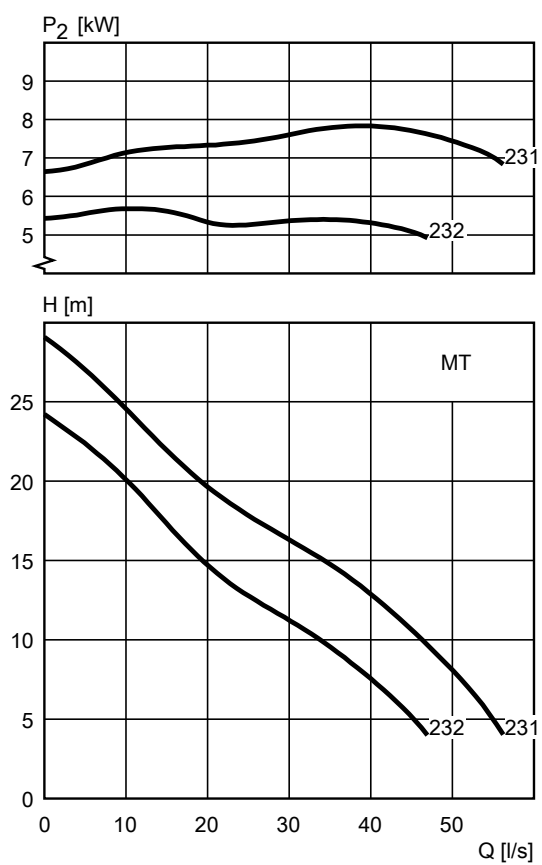
Рис. 17: MT, 50 ГД
