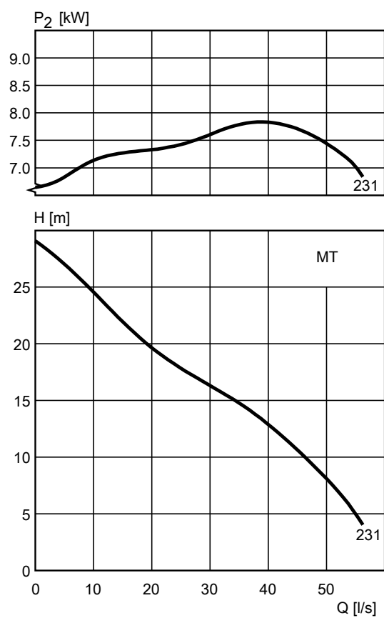
Рис. 13: МТ, 50 ГД
