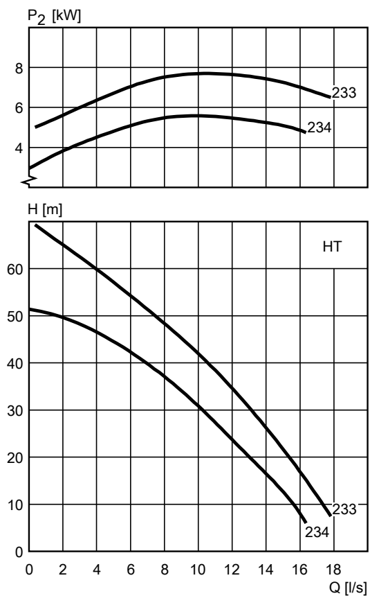
Рис. 15: HT, 50 ГП
