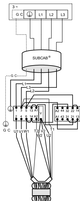
Соединение звездой
