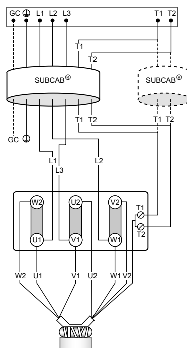
Соединение треугольником
