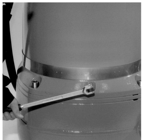
Рис. 20: С рубашкой охлаждения
