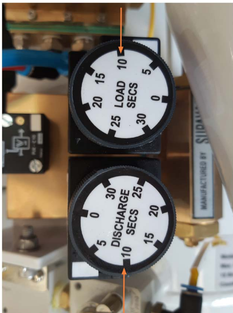
Рисунок 5 – Таймеры SV60V (кожух снят). Стрелками показаны ключевые точки для установки таймеров.
