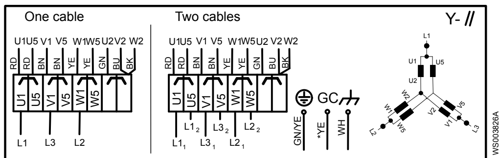
Рис. 11: параллельное соединение «звезда»
