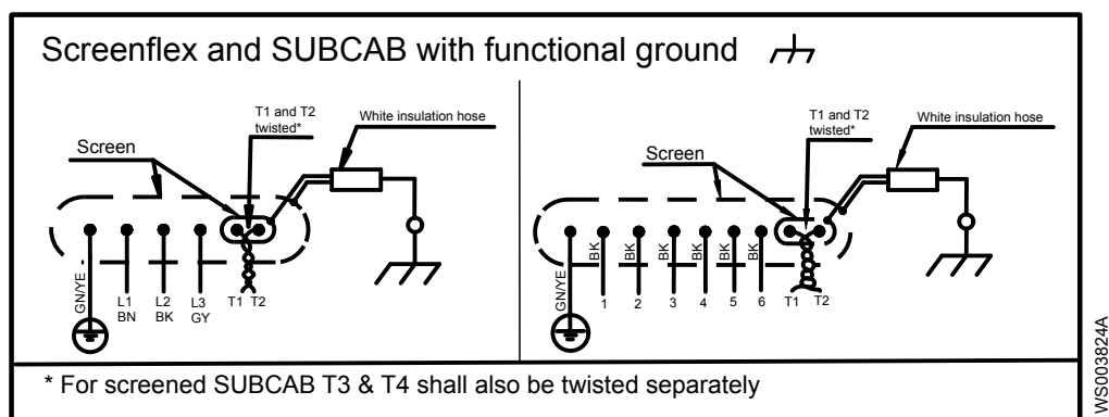
Рис. 14: Кабели Screenflex и SUBCAB с функциональным заземлением
