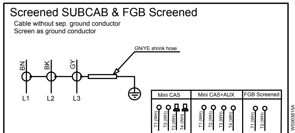
Рис. 13: Экранированный кабель SUBCAB и экранированный кабель FGB
