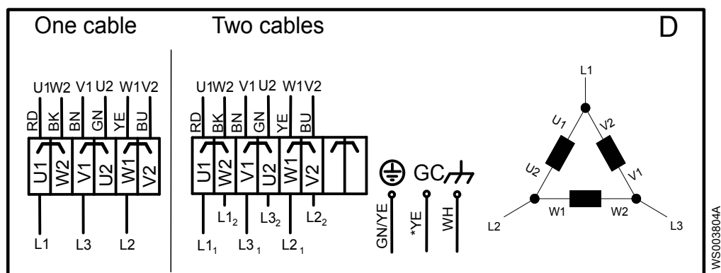
Рис. 8: «Треугольник»
