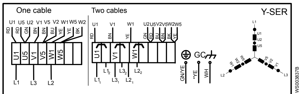
Рис. 12: последовательное соединение «звезда»
