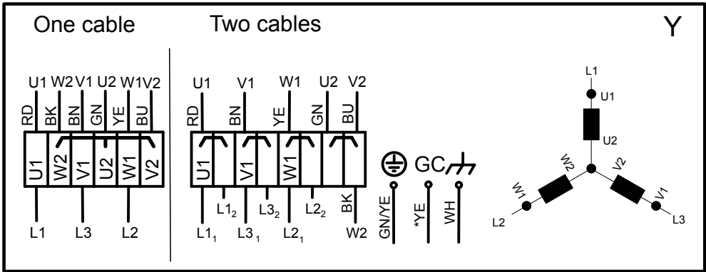
Рис. 7: Соединение "звездой"
