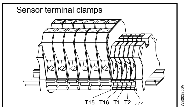
Рис. 16: Контактные зажимы датчика
