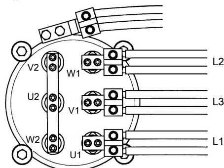
Рис. 32: Приводы 805/815, 835/845, 865/875, 885/895; 905/915, 935/945, 965/975; 705/715, 735/745, 765/775
