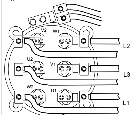
Рис. 34: Приводы 805/815, 835/845, 865/875, 885/895; 905/915, 935/945, 965/975; 705/715, 735/745, 765/775
