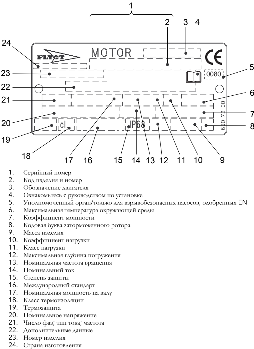
Рис. 8: Табличка для приводного блока начиная с 990101
