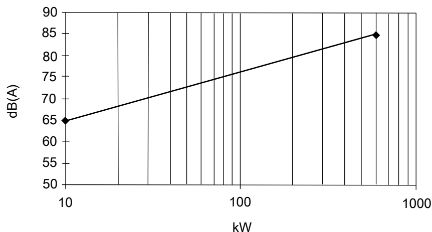
Рис. 40: Звуковое давление
