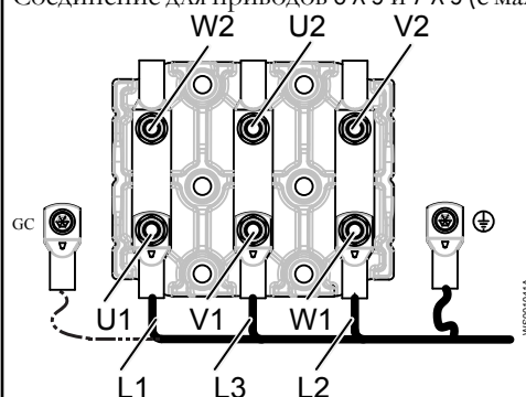
Рис. 25: Приводы 605/615, 665/675; 705/715, 735/745, 765/775
