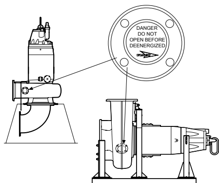
Рис. 12: Установка типа Т (слева) и установка типа Z
