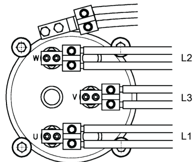
Рис. 23: Приводы 805/815, 835/845, 865/875, 885/895; 905/915, 935/945, 965/975; 705/715, 735/745, 765/775
