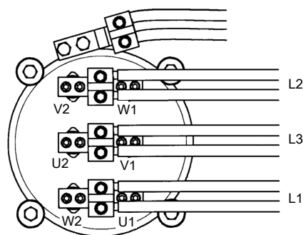
Рис. 28: 2 кабеля, приводы 805/815, 835/845, 865/875, 885/895; 905/915, 935/945, 965/975; 705/715, 735/745, 765/775
