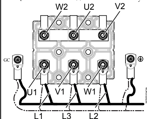
Рис. 31: Приводы 605/615, 665/675; 705/715, 735/745, 765/775
