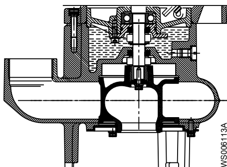
Рис. 11: Рабочее колесо типа C
