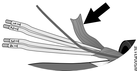
Рис. 7: Алюминиевая фольга на проводах цепей управления.
