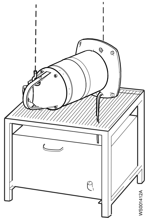
Рис. 15: Без рубашки охлаждения
