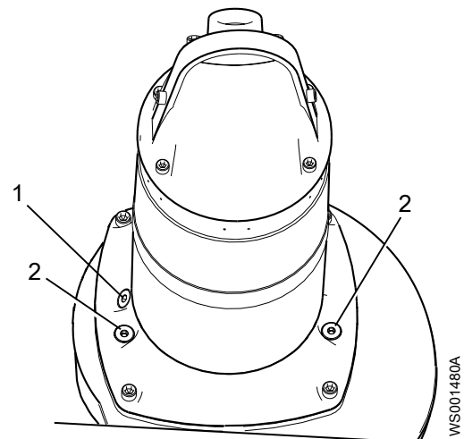
Рис. 11: Без рубашки охлаждения
