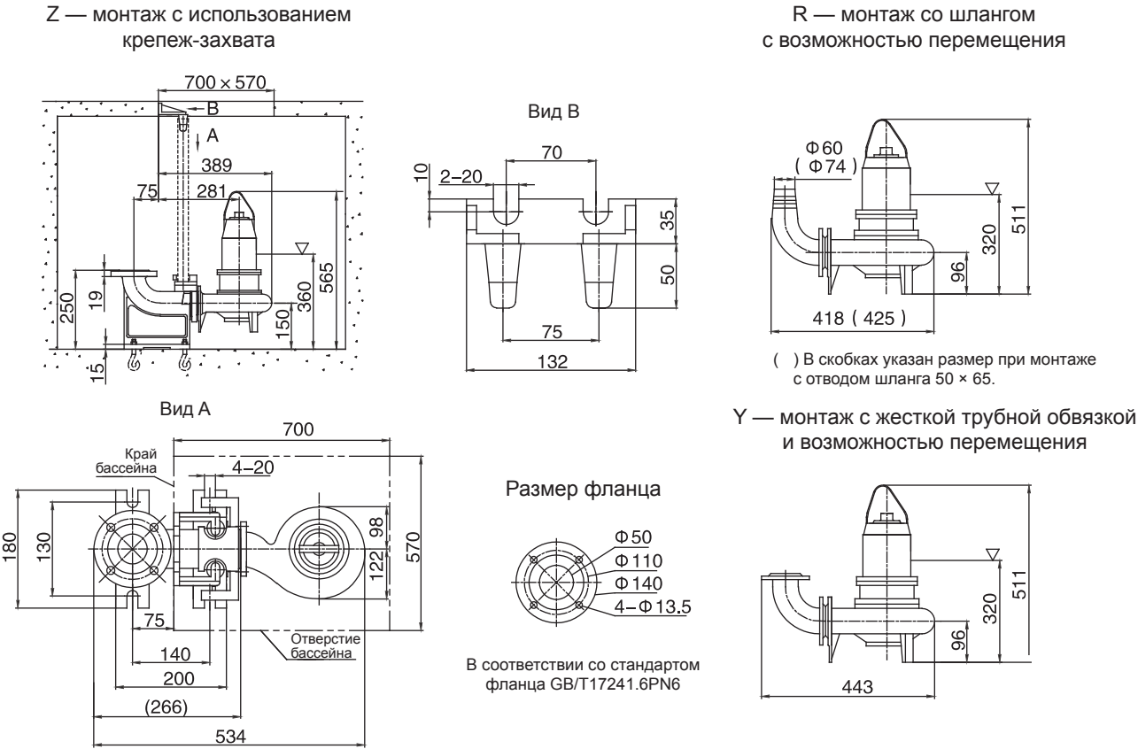
Монтажные размеры
