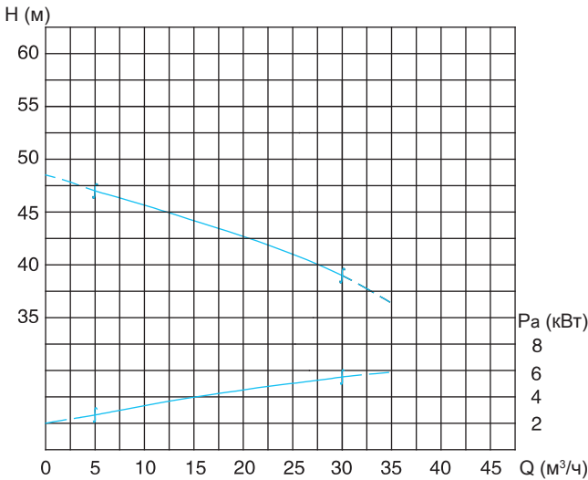
Кривая производительности
