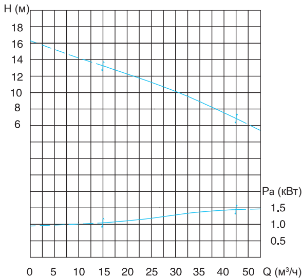
Кривая производительности
