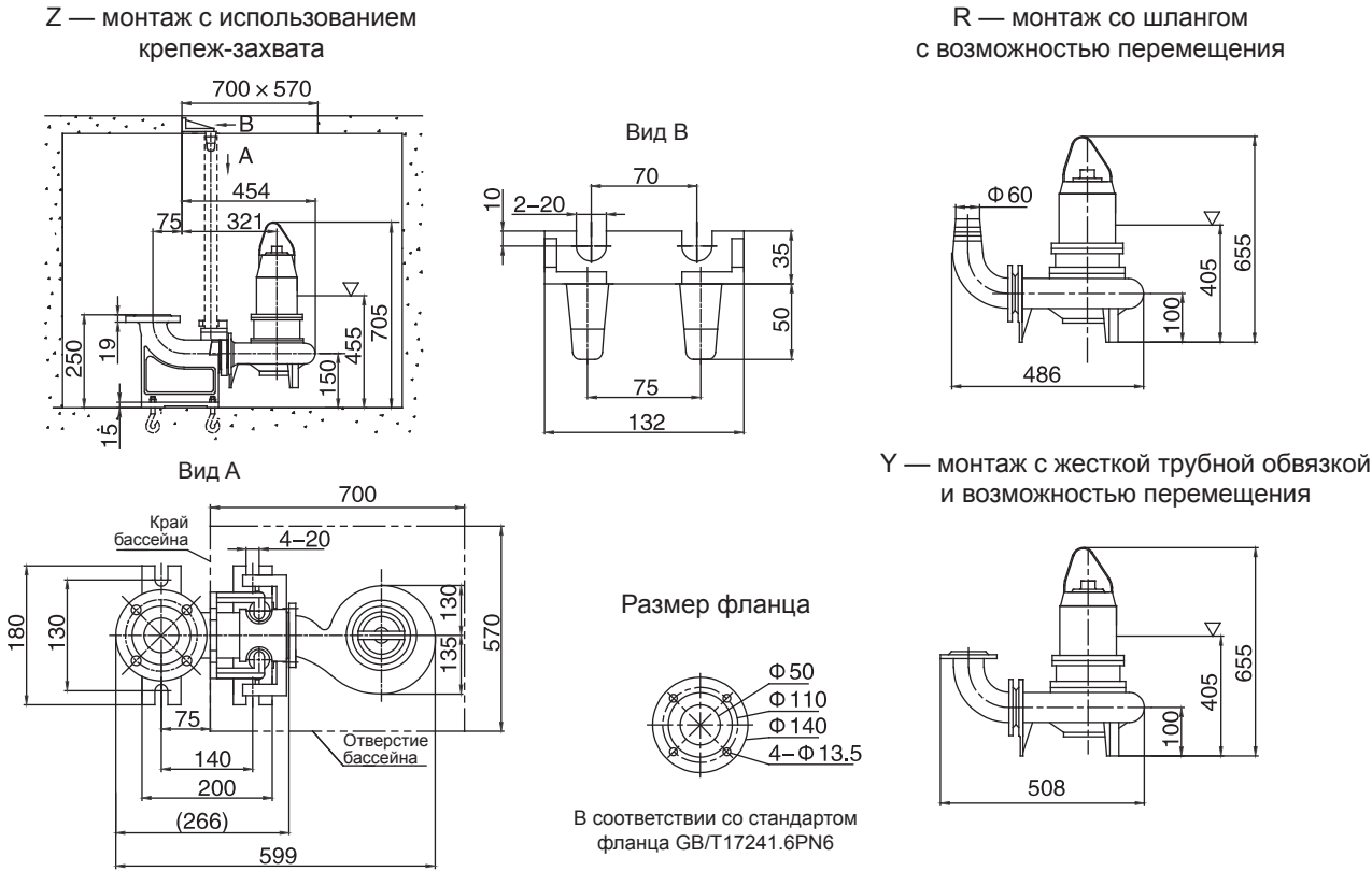
Монтажные размеры
