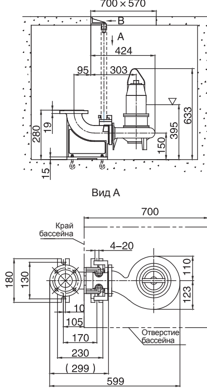
Z — монтаж с использованием крепеж-захвата
