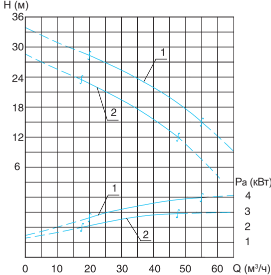
Кривая производительности
