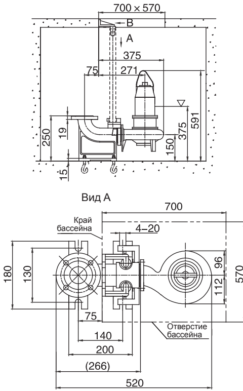
Z — монтаж с использованием крепеж-захвата
