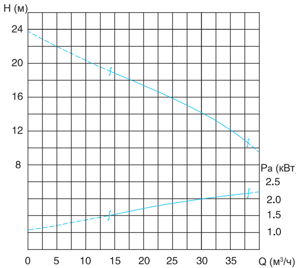
Кривая производительности
