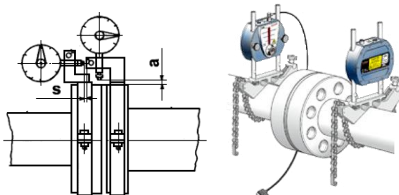
Индикаторное приспособление
