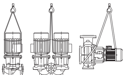
Рис. 7. Транспортировка насоса
