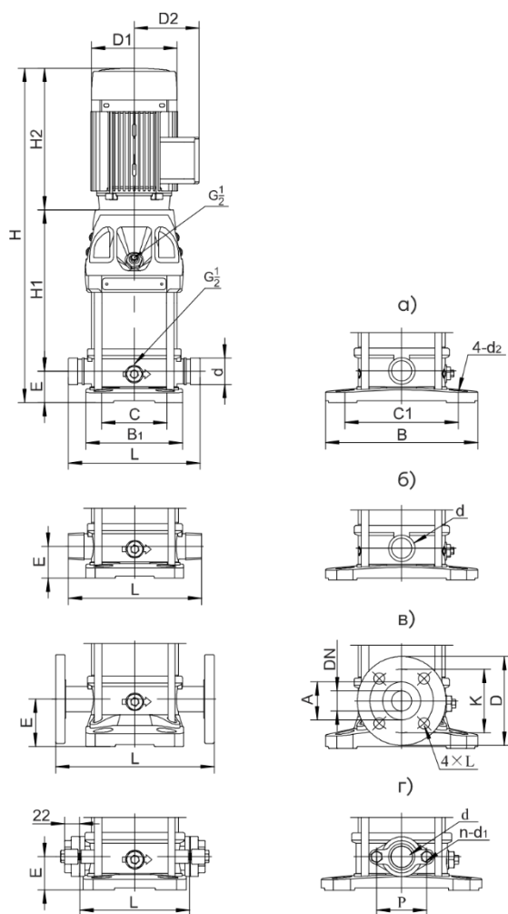
Рисунок 8 - Габаритно-присоединительные размеры а) vicaulic (гравлок); б) трубная резьба; в) DIN-фланец; г) овальный фланец
