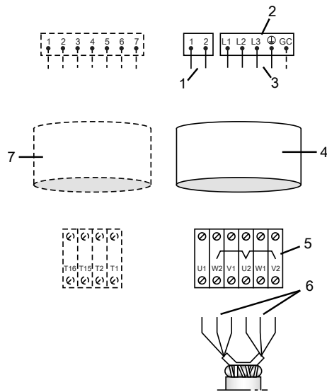
Рис. 7: Расположение подключений
