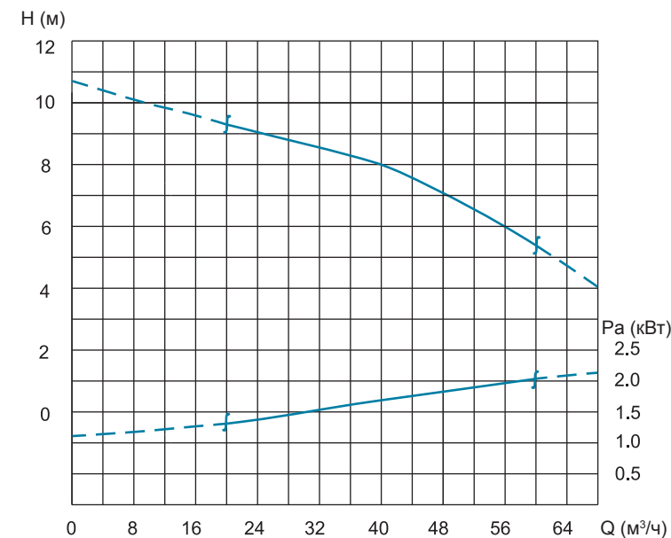
Кривая производительности
