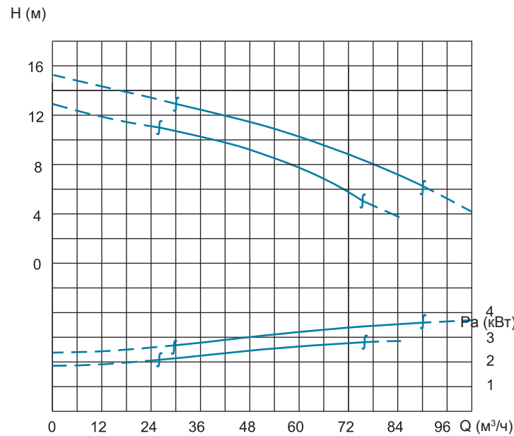
Кривая производительности
