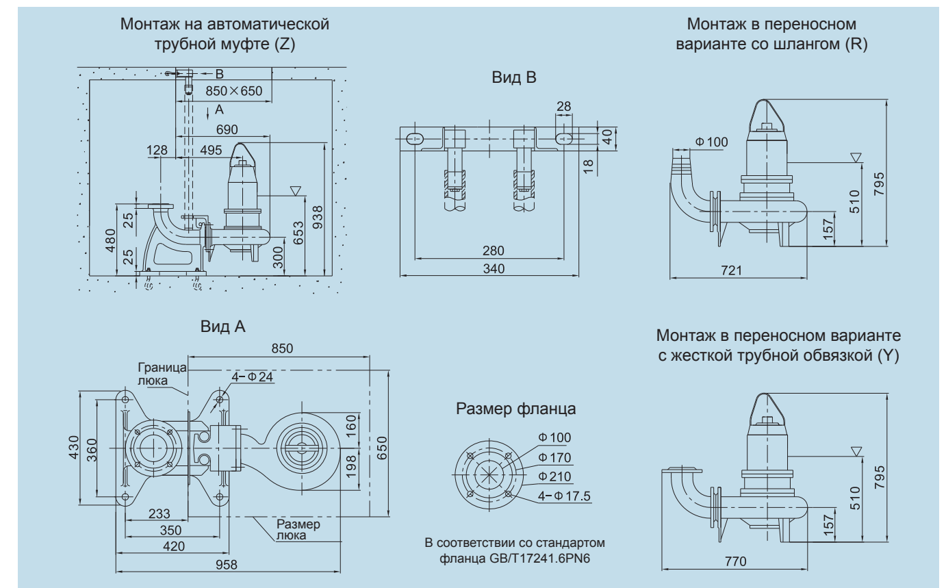
Монтажные размеры
