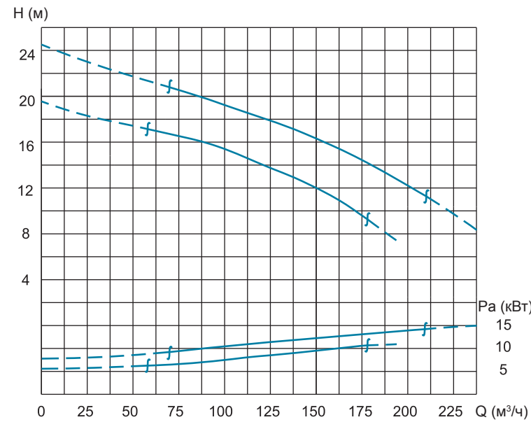
Кривая производительности
