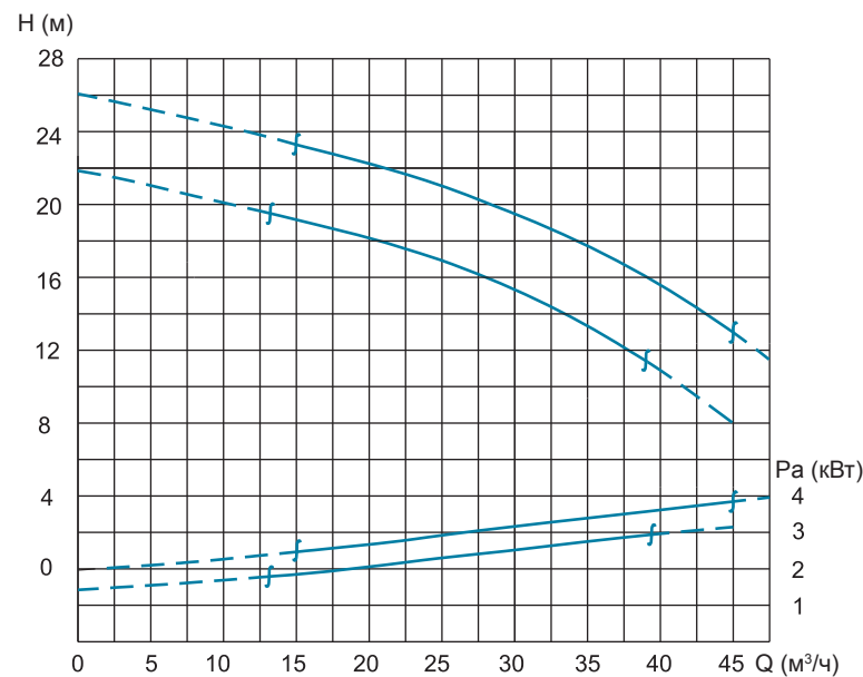
Кривая производительности
