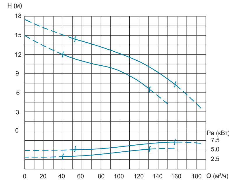
Кривая производительности
