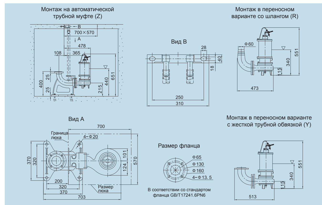
Монтажные размеры
