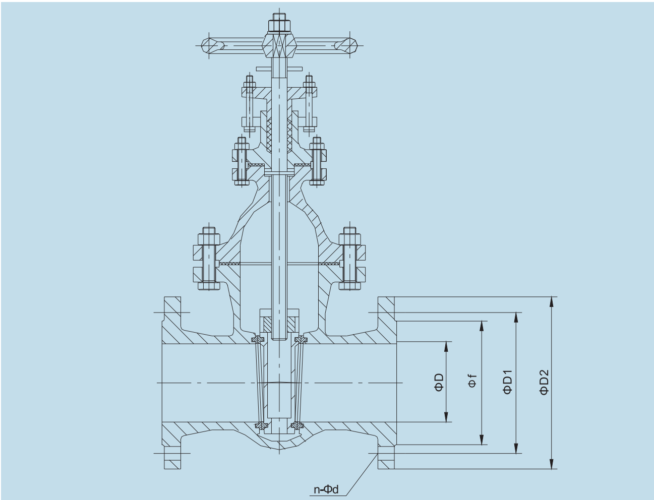
Задвижка
