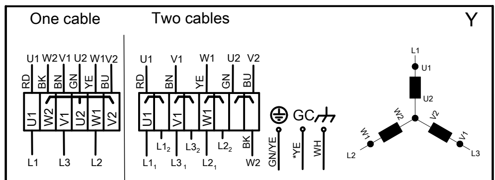
Рис. 14: Соединение “звездой”
