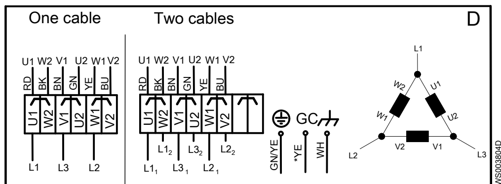
Рис. 15: «Треугольник»
