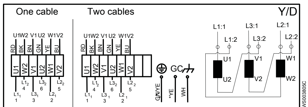
Рис. 16: «Звезда»/«Треугольник»
