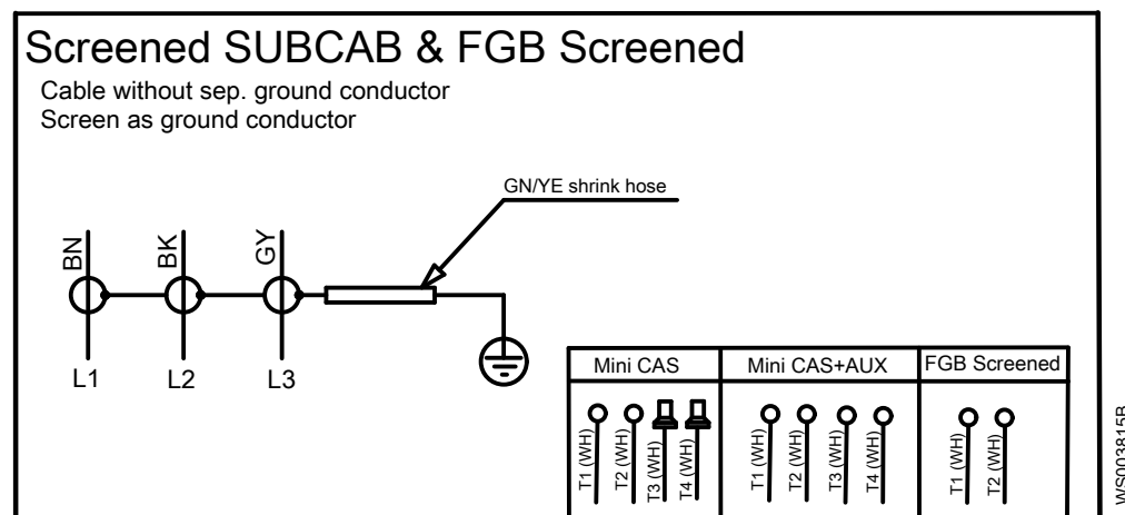
Рис. 20: Экранированный кабель SUBCAB и экранированный кабель FGB
