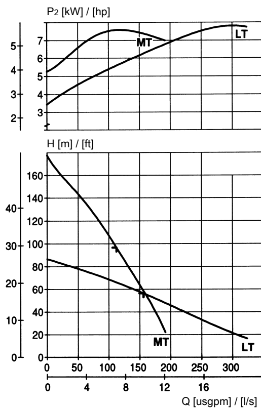
Рис. 6: 60 Гц, 3-фазный
