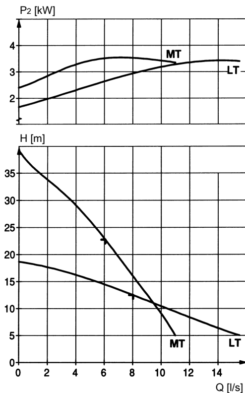
Рис. 4: 50 Гц, 3-фазный
