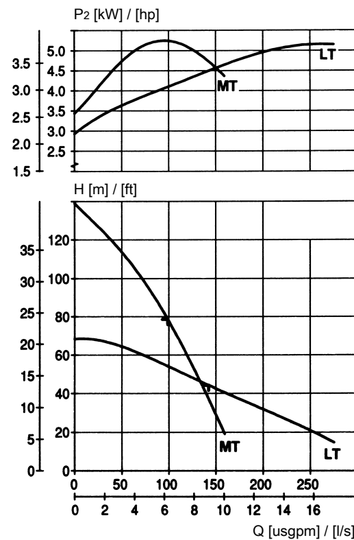
Рис. 5: 60 Гц, 1-фазный
