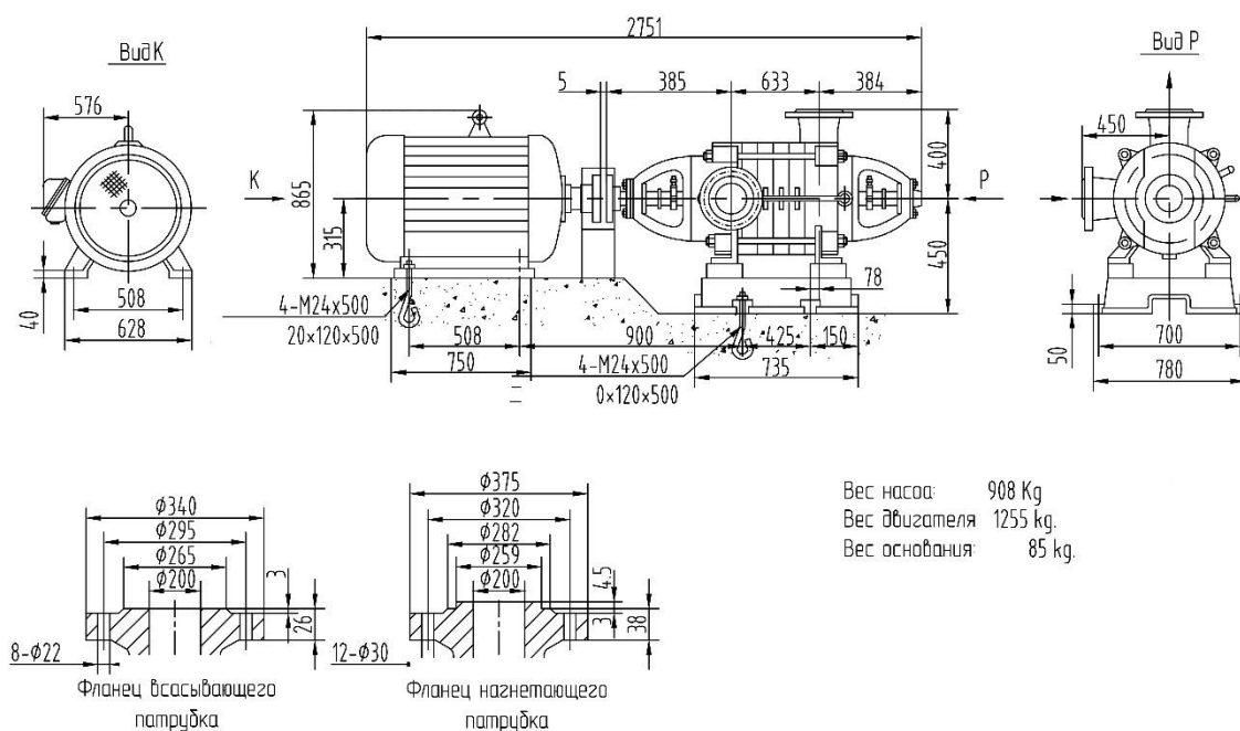
Габаритные размеры 200D43x4 I
