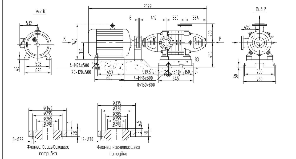
Габаритные размеры D360-40x3
