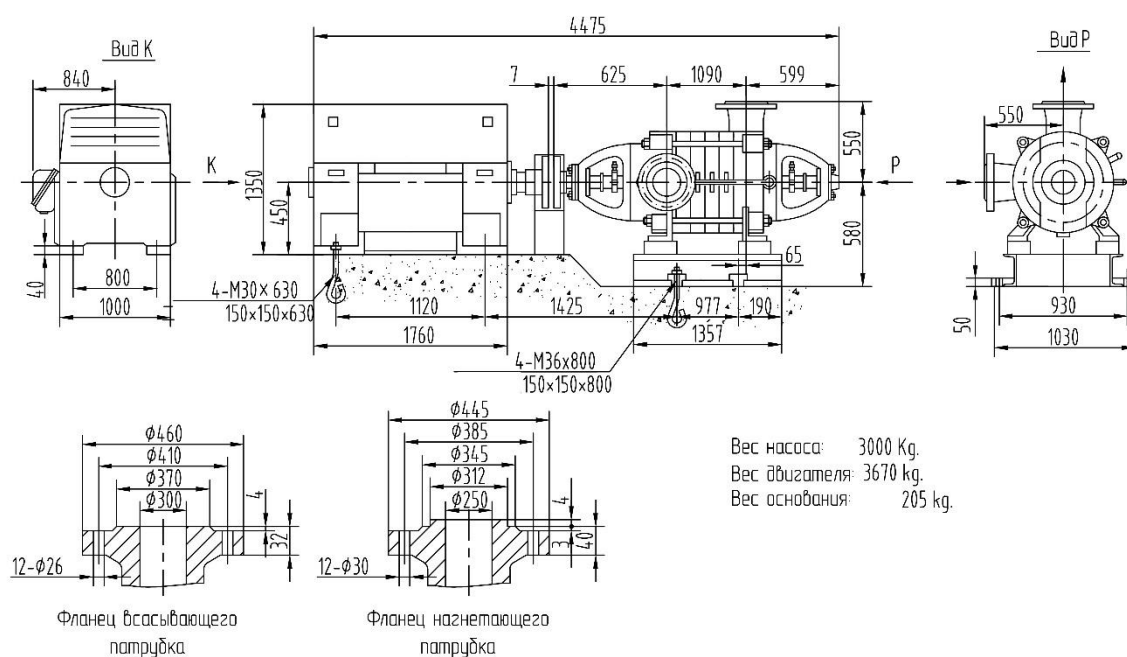
Габаритные размеры D600-60x5
