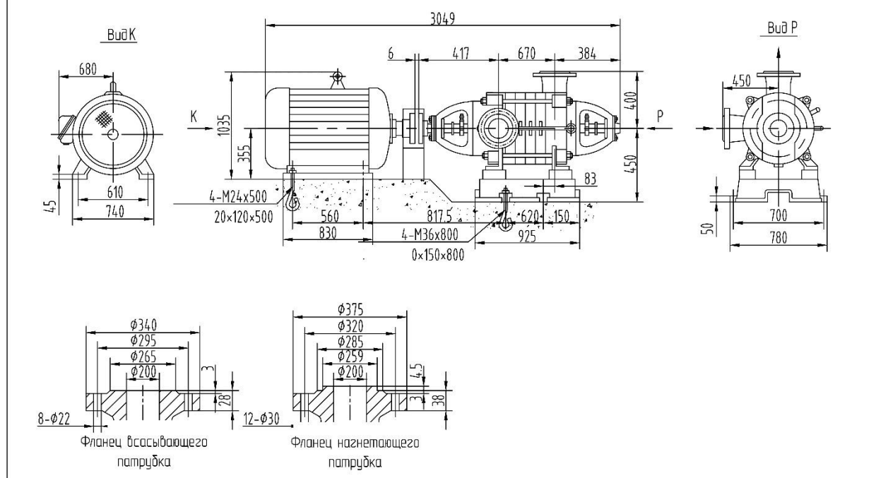
Габаритные размеры D360-40x4
