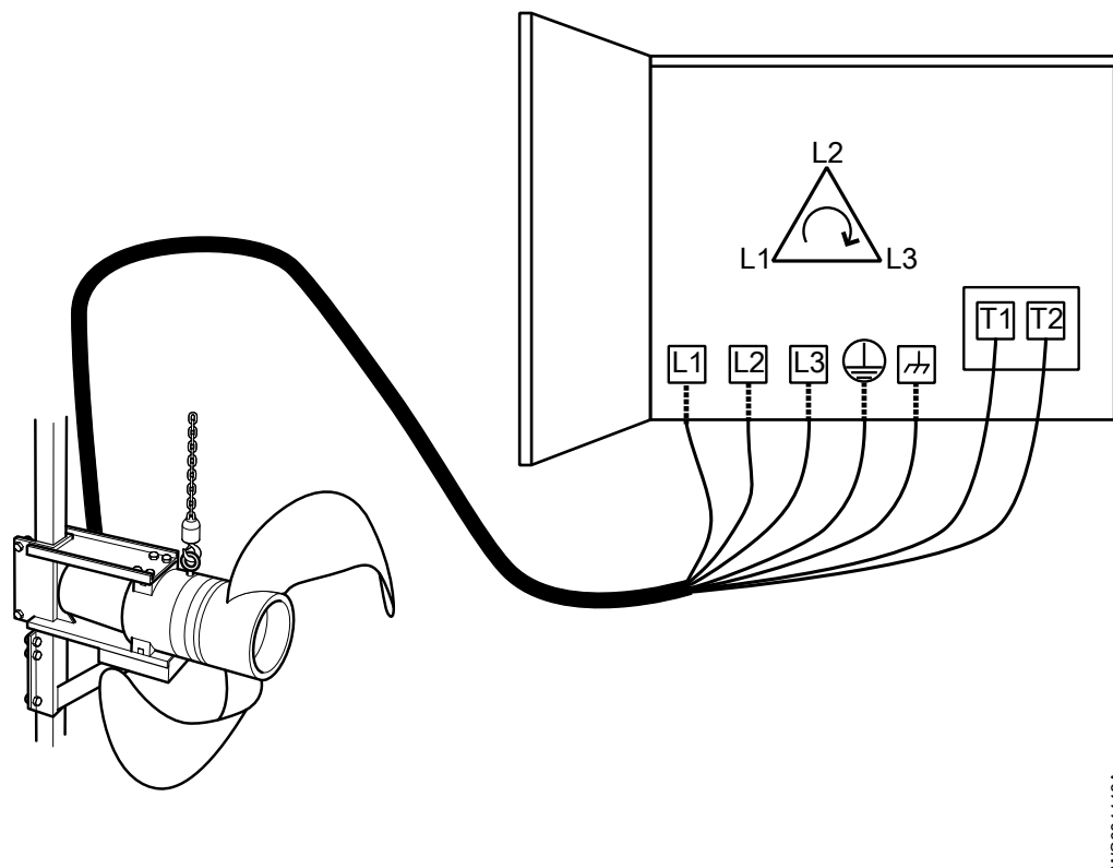
Рис. 5: Порядок чередования фаз
