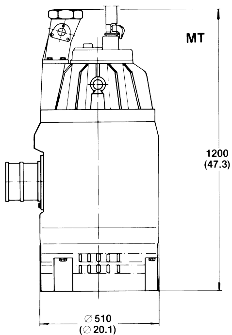
Рис. 14: MT
