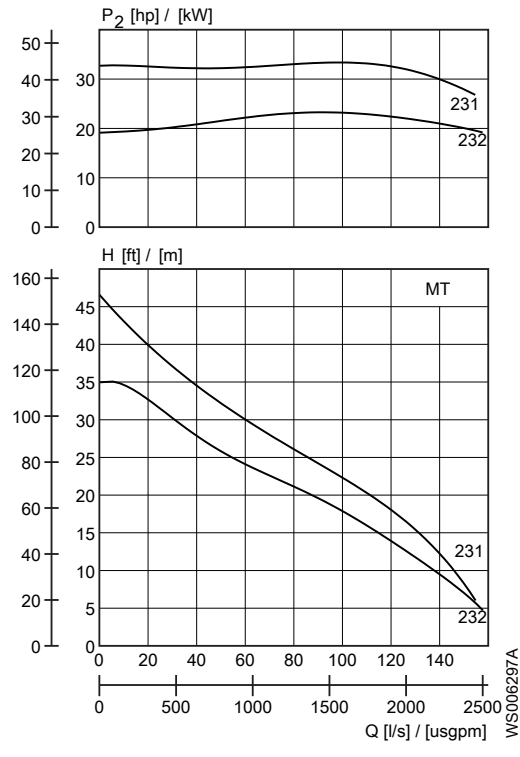
Рис. 23: 50 Гц, MT
