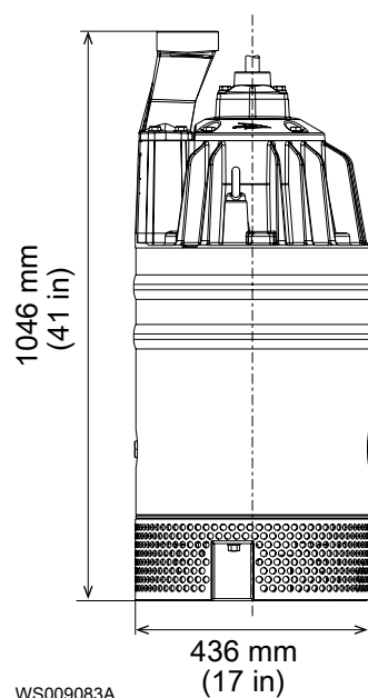
Рис. 12: HT
