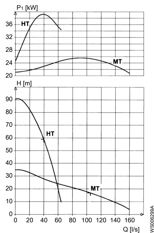
Рис. 26: 50 Гц, 37 кВт
