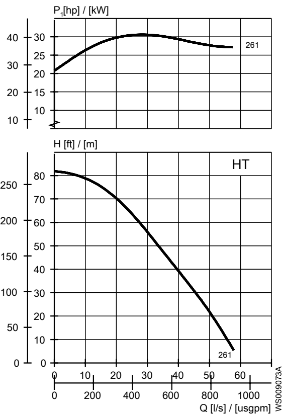
Рис. 17: 60 Гц, НТ
