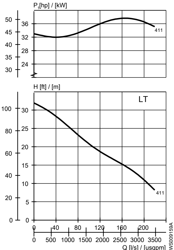
Рис. 21: 60 Гц, LT
