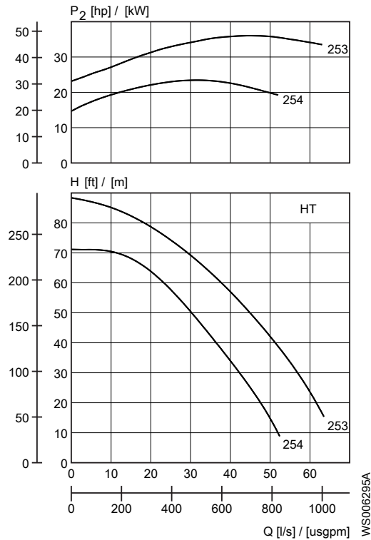
Рис. 22: 50 Гц, HT
