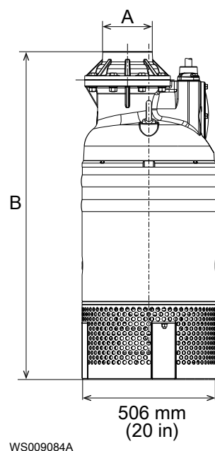
Рис. 13: LT, MT
