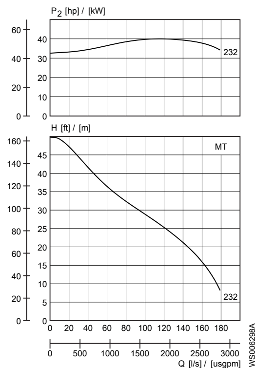
Рис. 25: 60 Гц, MT
