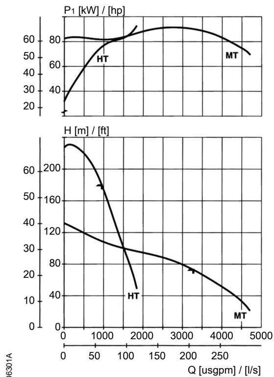
Рис. 6: 60 Гц, 1 770 об/мин
