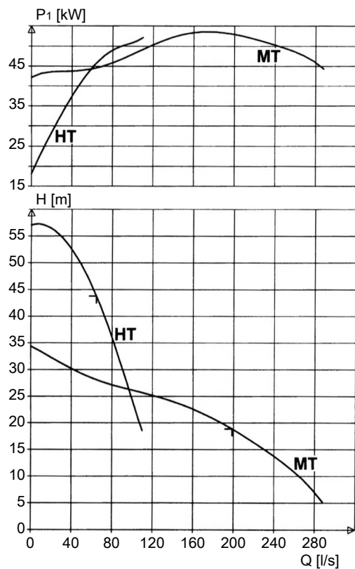
Рис. 5: 50 Гц, 1 470 об/мин
